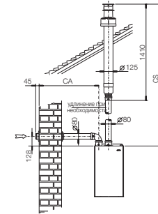
Раздельная система воздухозабора и вертикальным дымоотводом.
