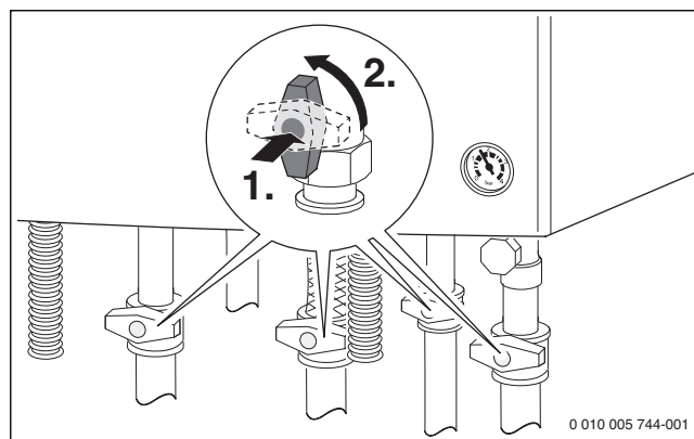
Рис. 2 Открытие сервисных кранов
